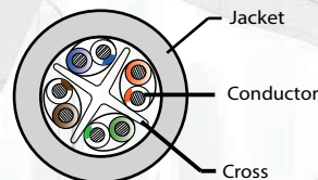
Cat 6 UTP
